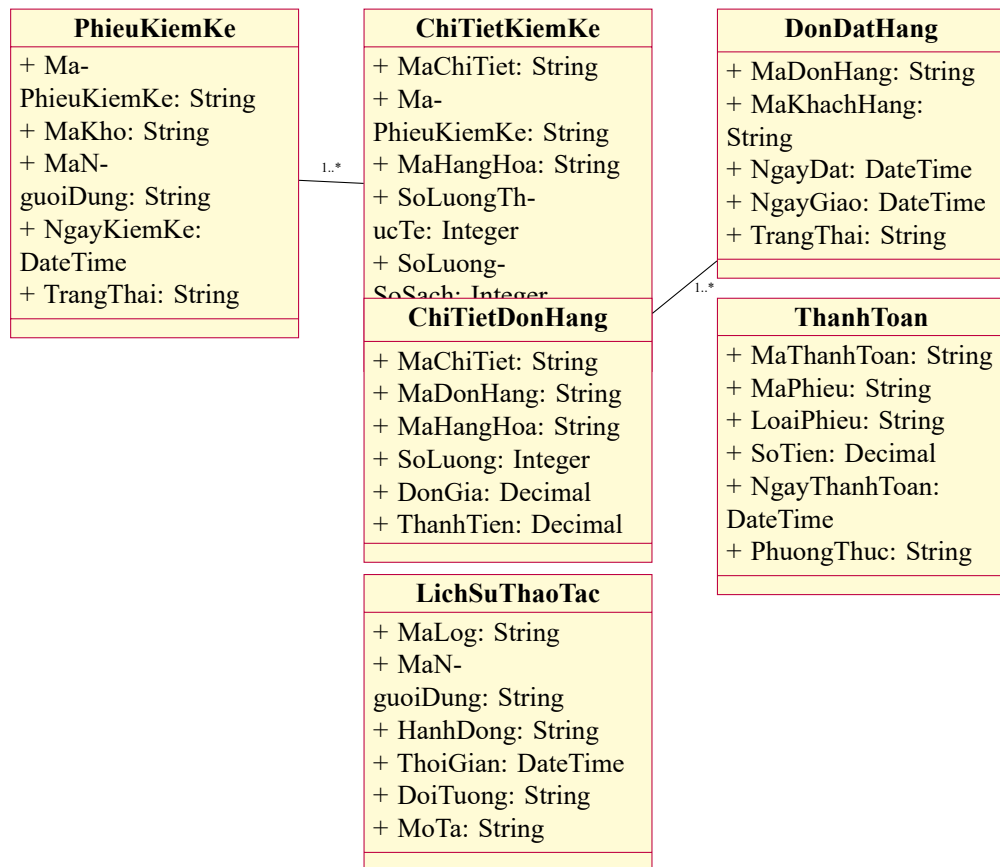
Hình 1: Sơ đồ lớp kiểm kê, đơn hàng và thanh toán
